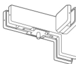
V564 Transom, side and interior fin panel link patch with pivot for double action doors. Pièce de jonction imposte et fixe latéral avec pivot et contre-ventement intérieur (cote penture) pour portes à double action.
