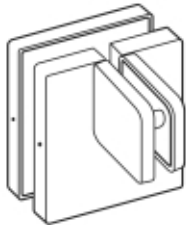
V585 Fixed panel connector with side and fin panel link patch. Liaison pour panneaux fixes avec ailette de contre-ventement.
