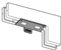
V521 Transom-side panel strike patch for corner lock. With or without stop. Pièce de jonction imposte et fixe latéral (cote poignée) avec gâche pour serrure d'angle. Avec ou sans butée.
